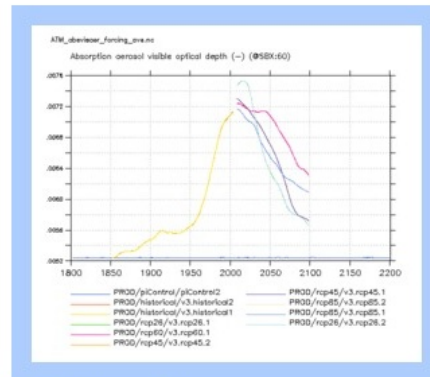
ATM_absvisae forcing_ave
