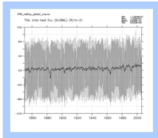
ATM_nettop_global
