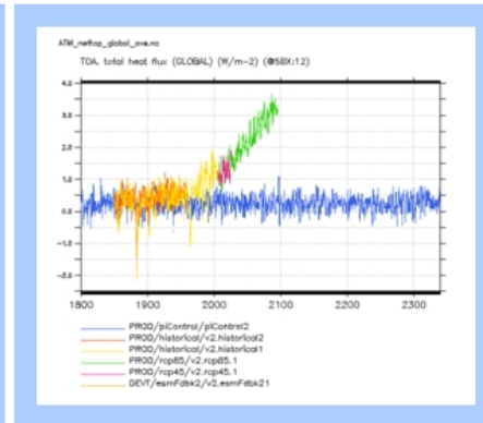
ATM_nettop_global_ave
