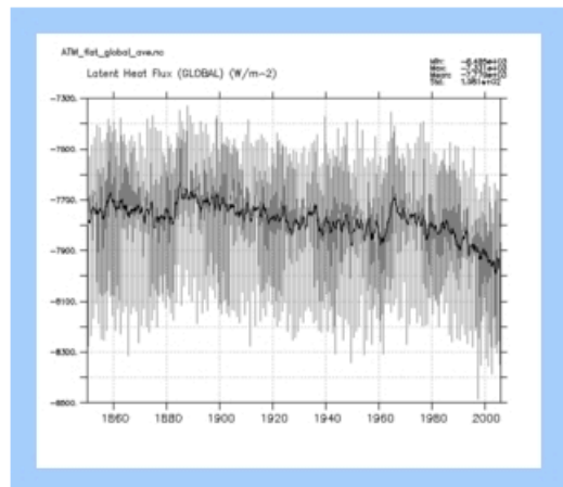
ATM_flat_global
