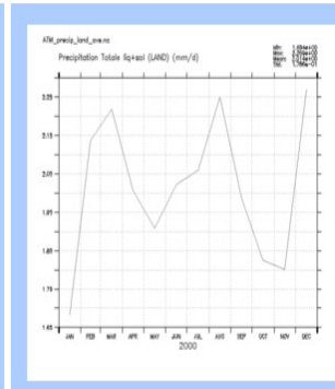
ATM_precip_land
