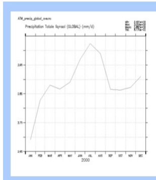
ATM_precip_global
