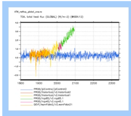
ATM_nettop_global_ave
