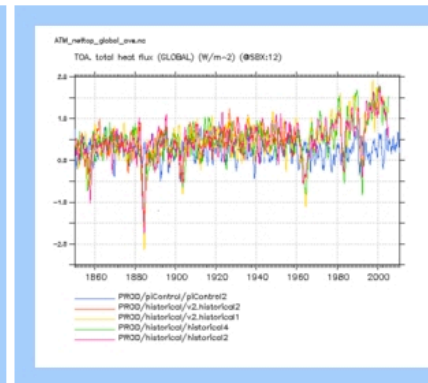
ATM_nettop_global_ave
