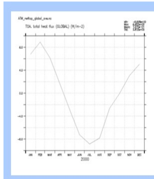
ATM_nettop_global
