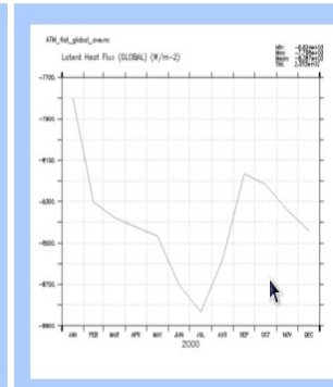
ATM_flat_global
